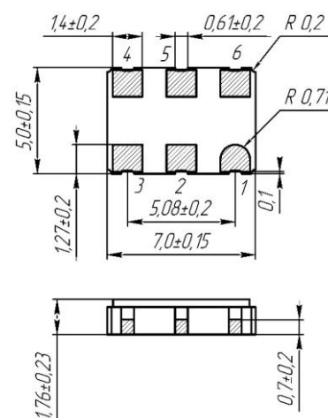
Корпус металлокерамический Покрытие площадок: Ni+Au(0,3...1 мкм)
